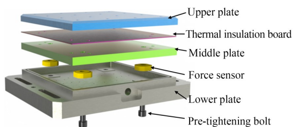
图2 测力仪结构
